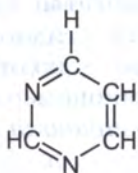
Пирими́дин
