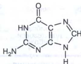
Гуа́нин
