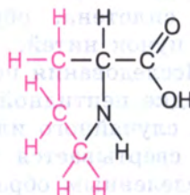
Пролин (про)
