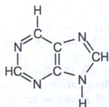
Пури́н
