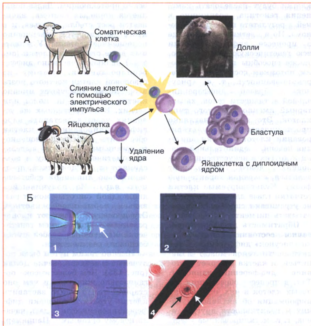
Рис. 135. Клонирование млекопитающих:
