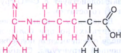
Аргинин (арг) *
