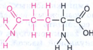
Глутамин (ггл)
