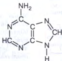
Аде́нин
