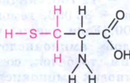
Цистеин (цис)
