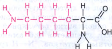
Лизин (лиз) *
