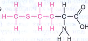
Метионин (мет) *
