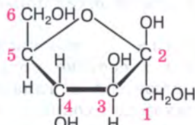
Фруктоза
